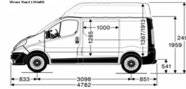
Vivaro Van L1 H1042
